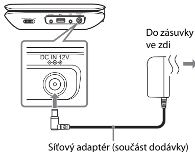
Síťový adaptér (součást dodávky)
