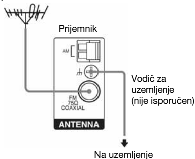
Vanjska FM antena
