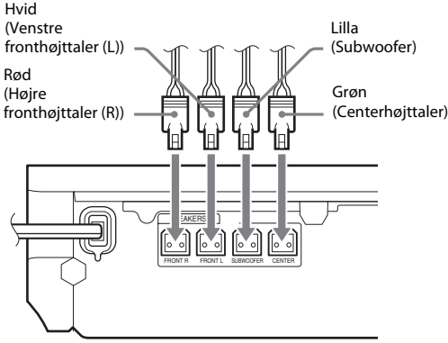
Enhedens bagpanel
