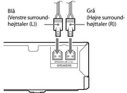
Surroundforstærkerens bagpanel
