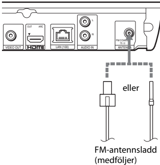
Enhetens bakpanel
