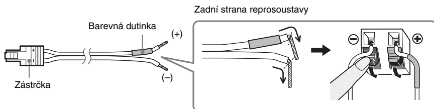
Zadní panel
