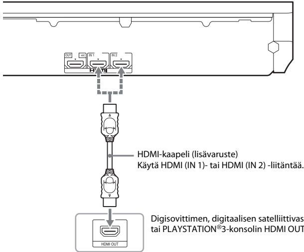
Laitteen takapaneeli
