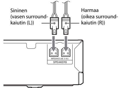
Surround-vahvistimen takapaneeli
