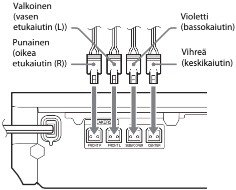
Laitteen takapaneeli
