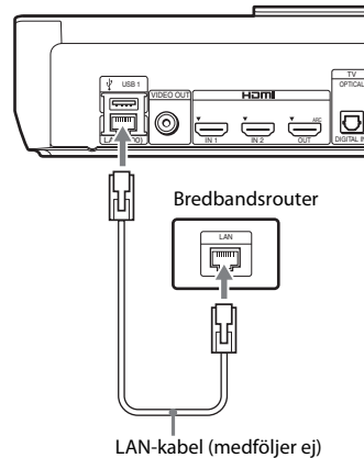
Enhetens bakpanel
