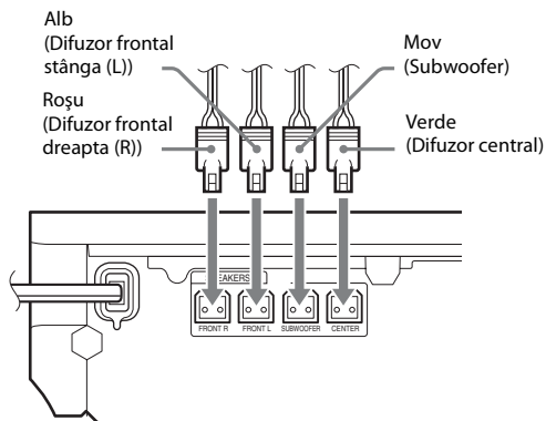
Panoul din spate al unității
