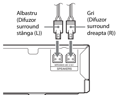
Panoul din spate al amplificatorului surround
