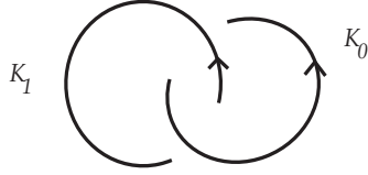
Fig. 2.1. The Hopf link.
