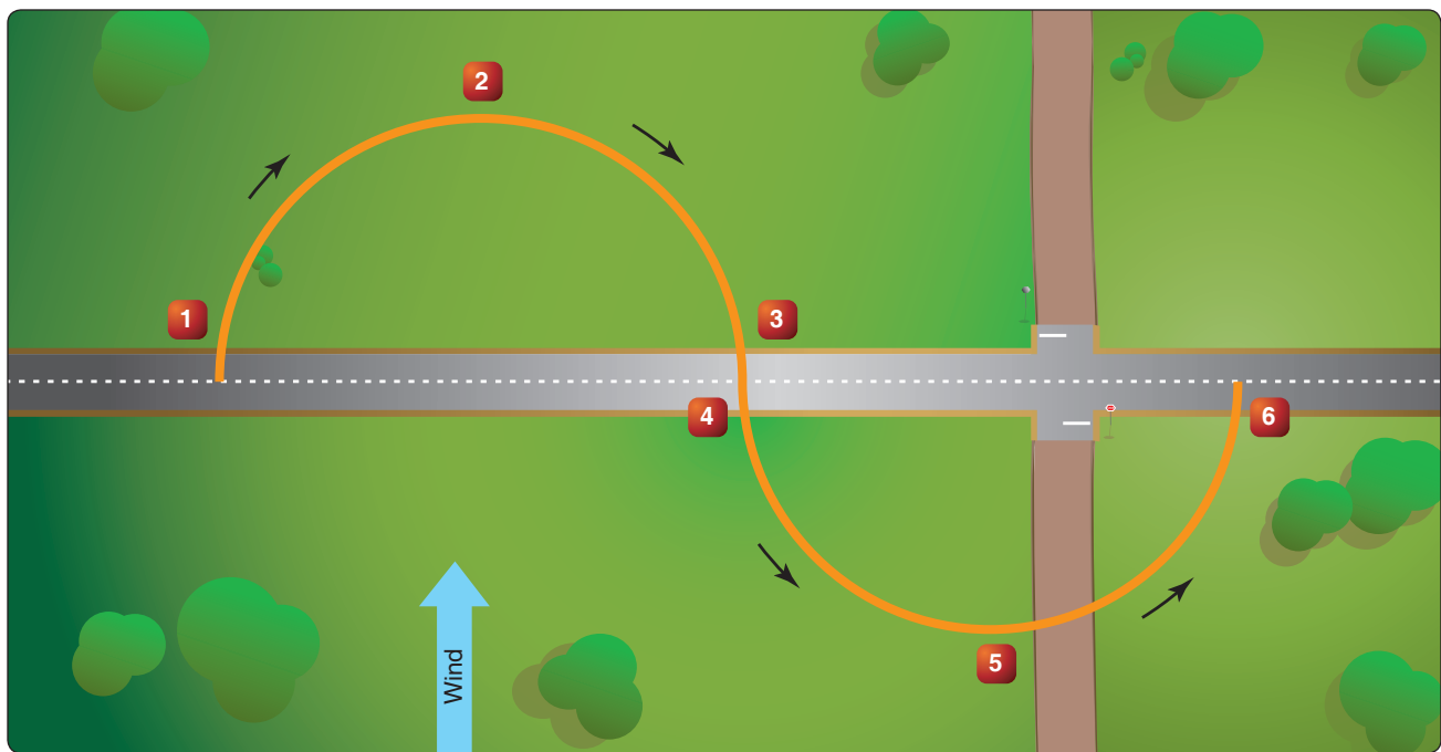
FIGURE 66.—S-Turn Diagram.
